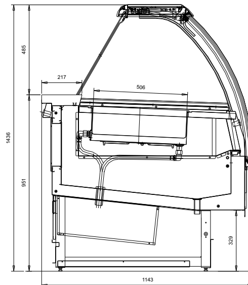
vetrina tavola calda bagnomaria
