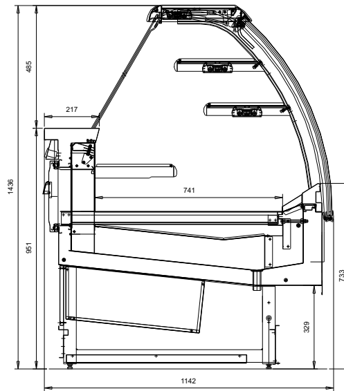
pasticcera - con cassetti
